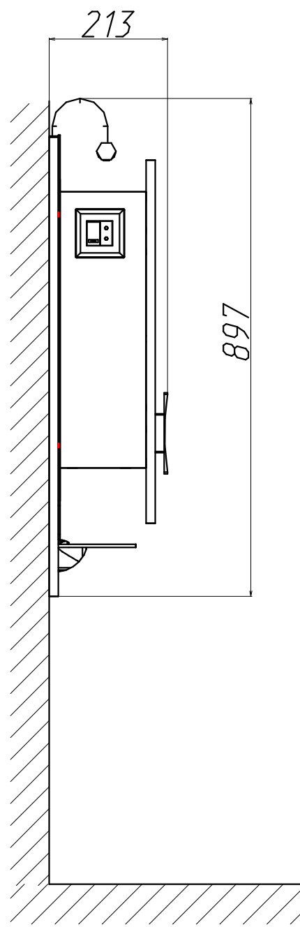
Н - Крепления навесок; Э - точка вывода электропровода; В - желаемая высота
